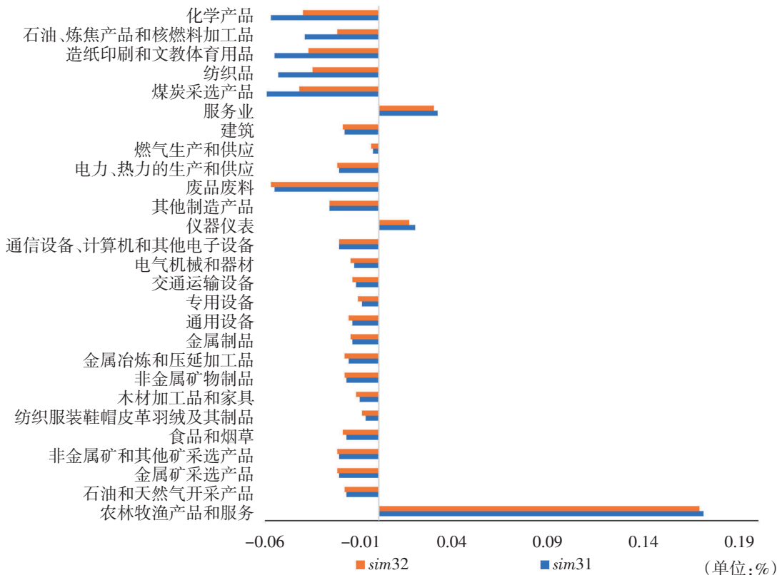
图4 征收惩罚性水价对不同产业用水量的影响 ( k=m, h, s )
